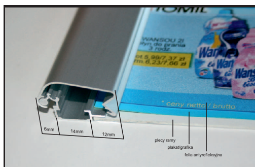
Na zdjęciu przekrój profilu OWZ P3.
